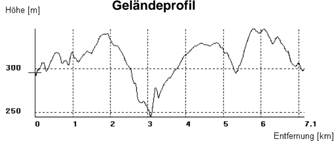
Geländeprofil
